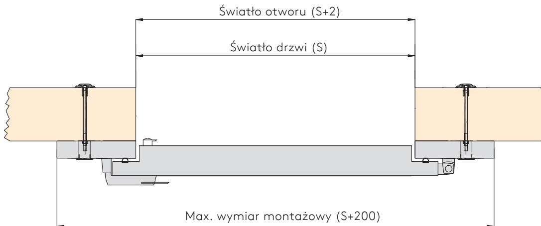
Montaż do płyty - futryna jednostronna
